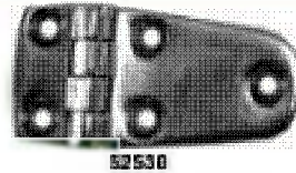
52530 : HINGE ( C.P.B. ) Size : 57 x 38 mm.
